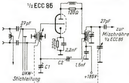
Bild 1. UKW-Eingangsstufe für Rundfunkempfänger mit FM- Z_f = 6,75 \text{ MHz} ; man beachte die „gemischte“ L- und C-Abstimmung (C1 = Abgleichstrimmer für den Eingangskreis, C2 = Trimmer für die Neutralisation)
