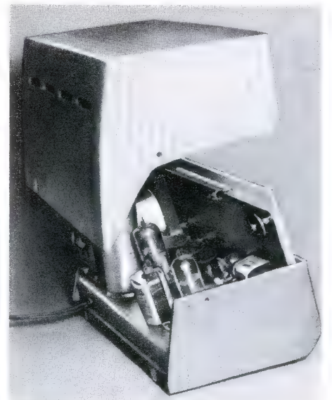
Bild 3. Aufbau des Chassis und der Haube bei Anwendung der modernen Form
