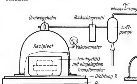
Bild 1. Die Entwicklung für die Vakuumtränkung
