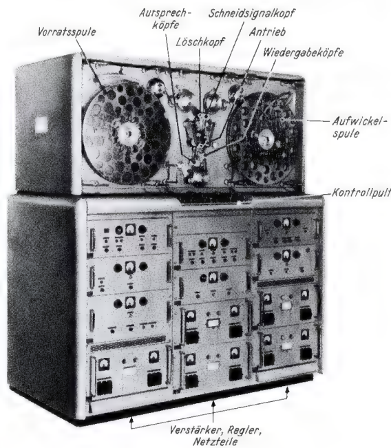
Rechts: Bild 1. Videosignal-Aufzeichnungsmaschine Vera der BBC-London mit einer Bandgeschwindigkeit von 508 cm/sec und einer Aufzeichnungsdauer von 15 Minuten. Mit zwei Maschinen, die von einem gemeinsamen Steuerpult aus bedient werden, ist pausenlose Aufnahme bzw. Wiedergabe möglich
