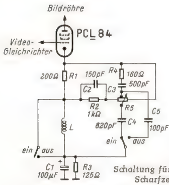
Bild 3. Schaltung für Weich- und Scharfzeichnung
