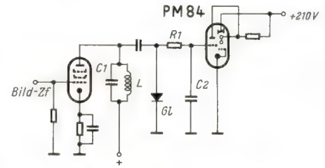
Bild 11. Prinzipschaltung der Abstimmanzeige mit dem Magischen Band
