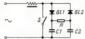
Schaltung zur Funkenlöschung für den Schalter S
