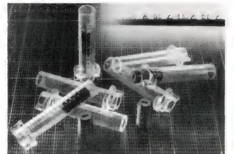
Bild 1. Der neue Spulenkörper weist einseitig nur eine schmale Gewindeleiste auf, die einen weich und elastisch wirkenden Spielausgleich zwischen Gewindekern und Halterung ohne Verwendung eines zusätzlichen Bremsmittels (Gummifaden, Kunststoffstreifen o. ä.) ermöglicht
